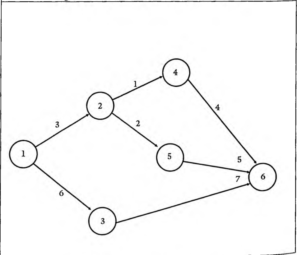
Figura 11.12b Cuadro de actividades, secuencias, red
