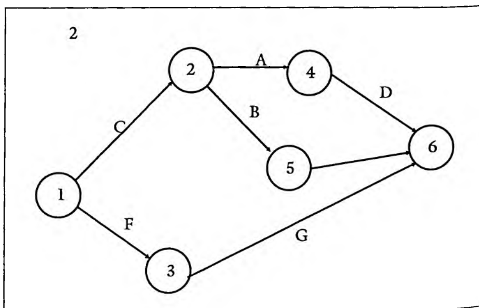
Figura 11.11 Red de actividades
