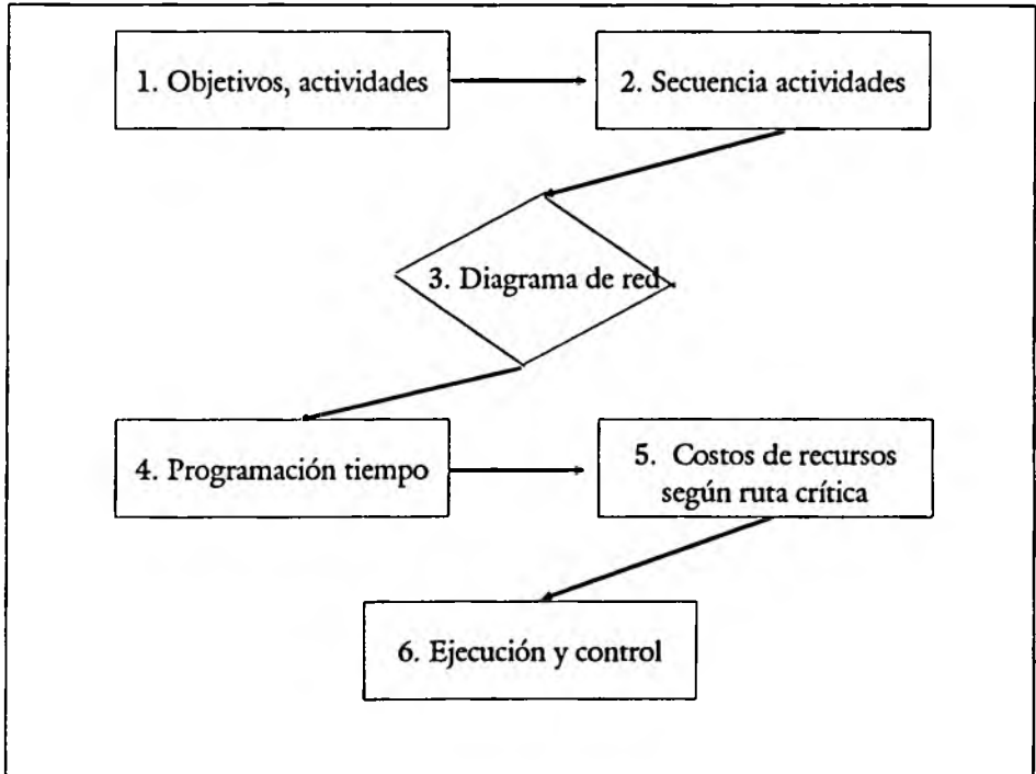
Figura 11.6 Pasos en la aplicación del Pert-CPM
